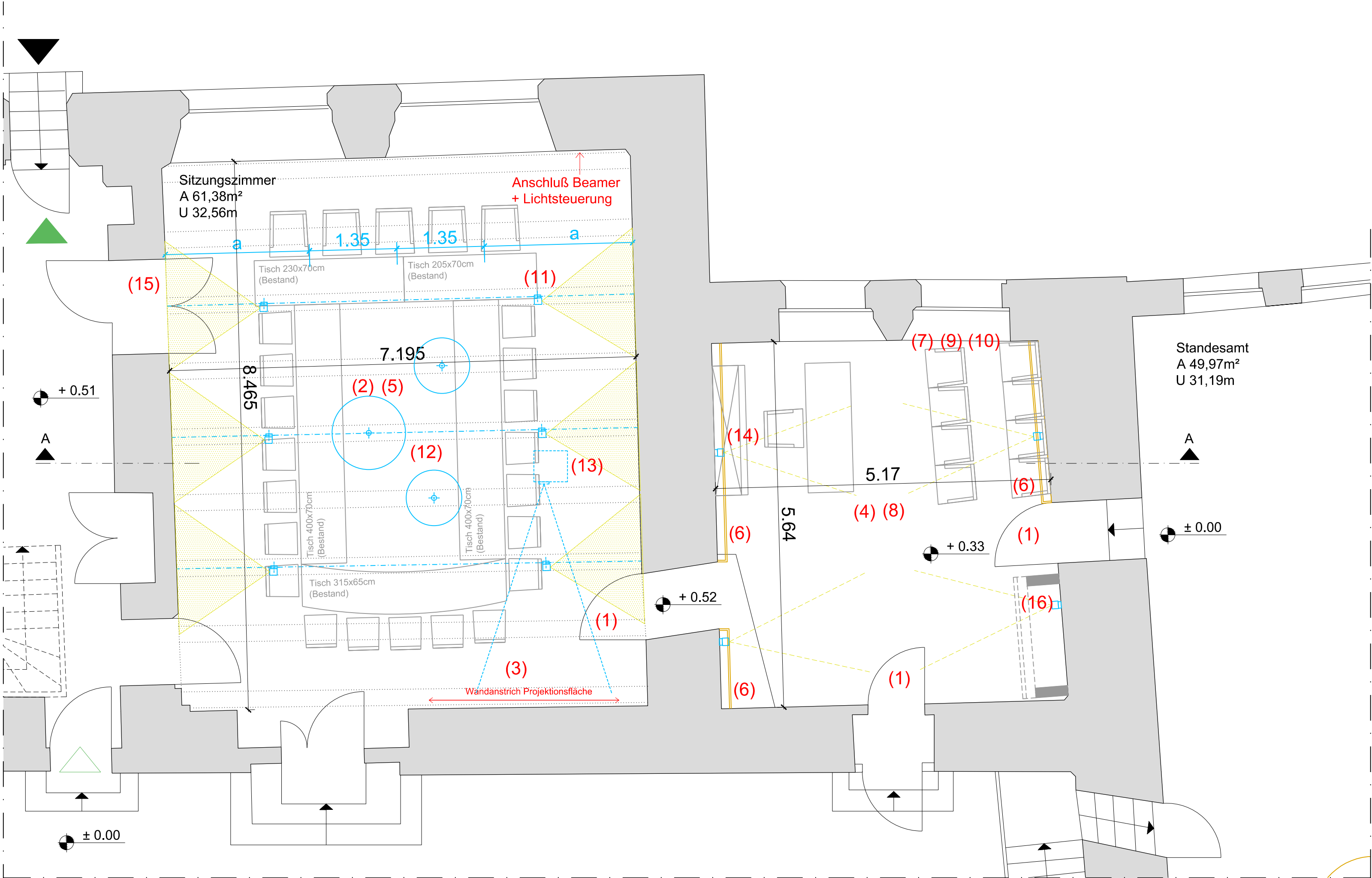
Grundriss
