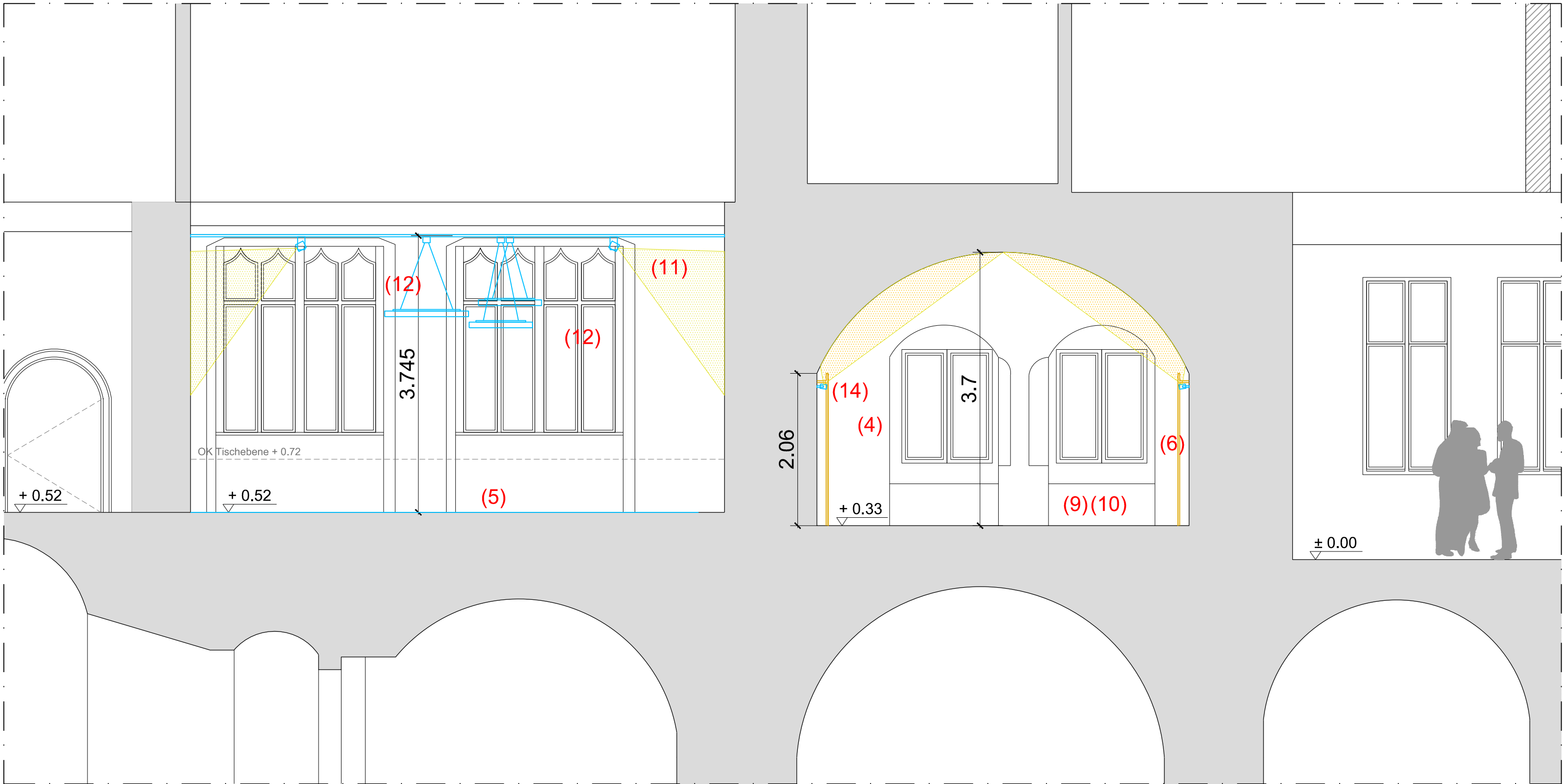
Schnitt A-A
